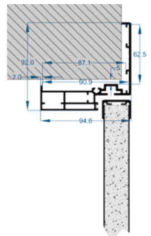
Coupe verticale
